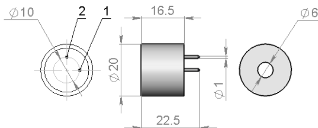
Рис.1 Размеры сенсора и схема расположения выводов 1 - индикаторный электрод 2 - вспомогательный электрод
