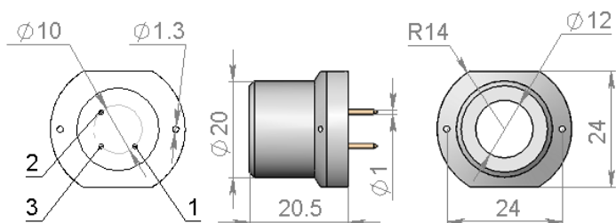
Рис.1 Размеры сенсора и схема расположения выводов
