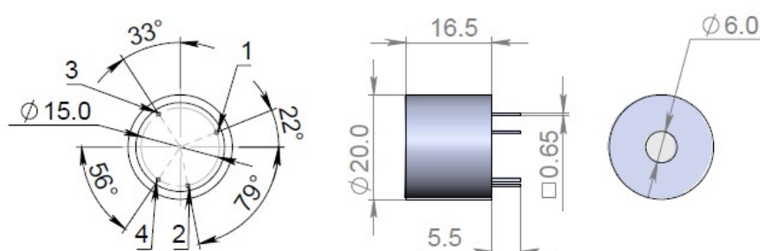
Рис.1 Размеры сенсора и схема расположения выводов
