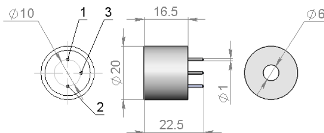
Рис.1 Размеры сенсора и схема расположения выводов
