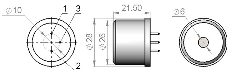
Рис.1 Размеры сенсора и схема расположения выводов 1 - индикаторный электрод 2 - вспомогательный электрод 3 - электрод сравнения
