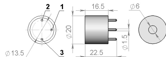
Рис.1 Размеры сенсора и схема расположения выводов 1 - индикаторный электрод 2 - электрод сравнения 3 - вспомогательный электрод
