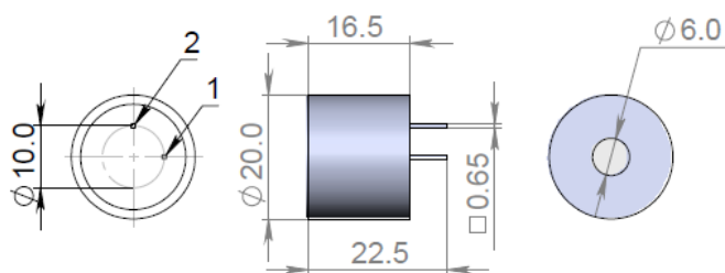
Рис.1 Размеры сенсора и схема расположения выводов 1 - индикаторный электрод 2 - вспомогательный электрод
