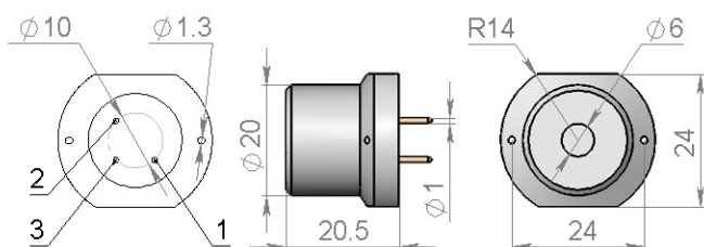
Рис.1 Размеры сенсора и схема расположения выводов 1 - индикаторный электрод 2 - вспомогательный электрод 3 - электрод сравнения
