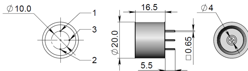
Рис.1 Размеры сенсора и схема расположения выводов
