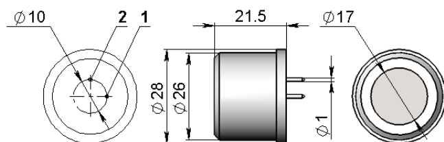
Рис.1 Размеры сенсора и схема расположения выводов
