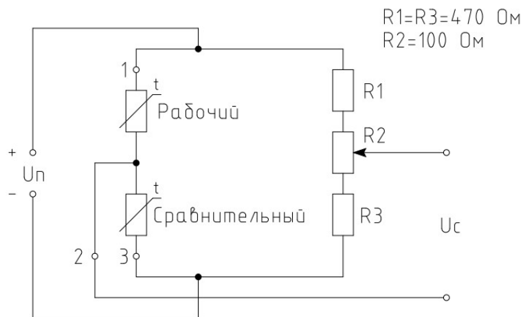
Рис.2 Включение сенсора в мостовую схему (рекомендуемое).
